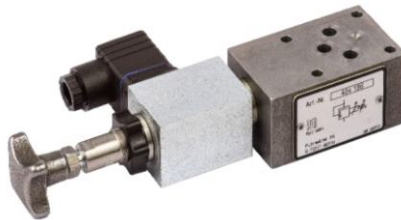
Parça Adı: Output regulation, prop. 24V
