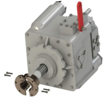
Parça Adı: Hydraulic pump 90cc
